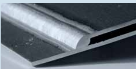
Saldatura AC-MIG con VARIGON® He15S su lamiera di spessore 1 mm e gap 1,5 mm
